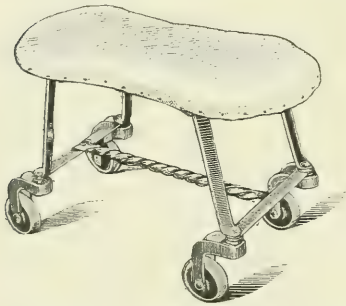
Fig. 125 a. LORENZsches Ruderbänkchen. (Verfertigt von L. Baumann, Wien.)
